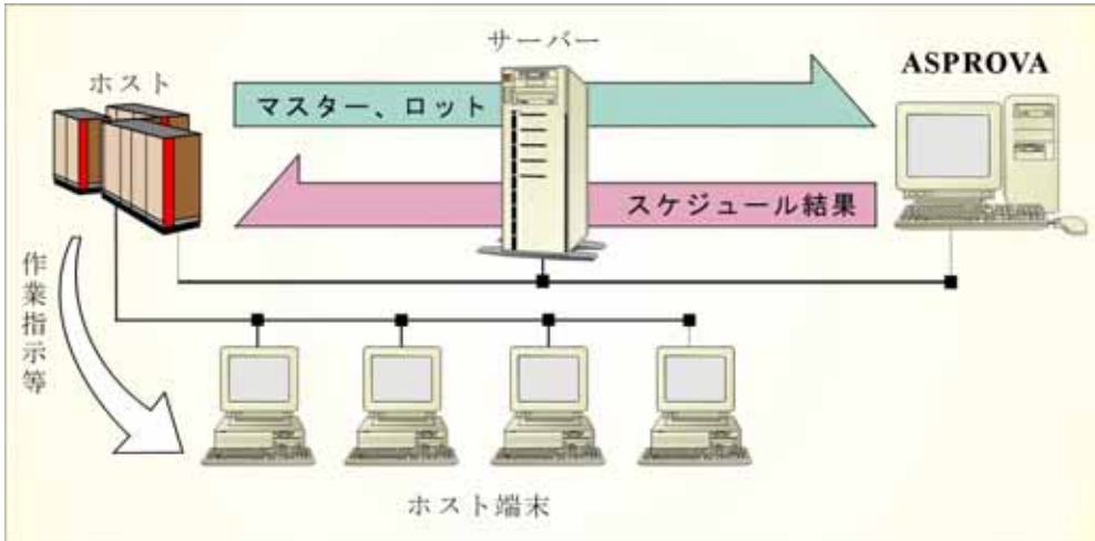
図1：システム構成図 ホストからサーバー経由でASPROVAにデータが送信される。ASPROVAからはスケジュール結果を返し、ホストから各工程にあるホスト端末に製造指示等が送られる。
